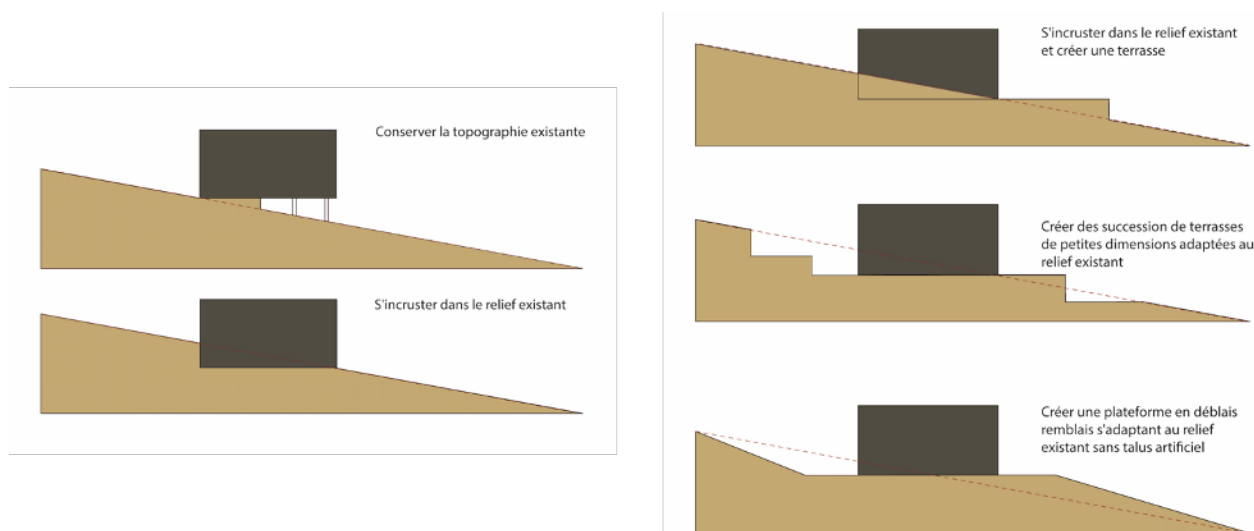
Schéma opposable d'implantation et d'adaptation du bâti
